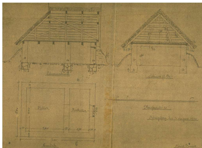
Plan piwnicy, widok i przekrój
