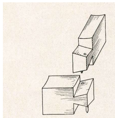
Złącze ciesielskie na „jaskółczy ogon”
