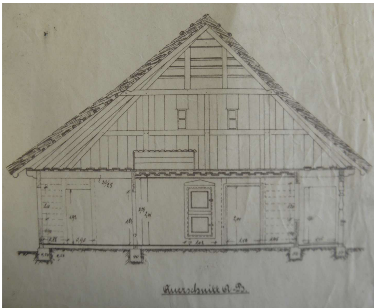
Przekrój poprzeczny
