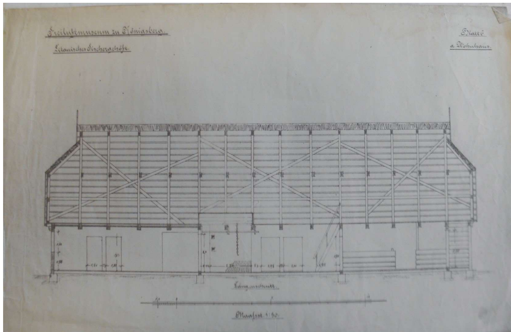
Przekrój podłużny
